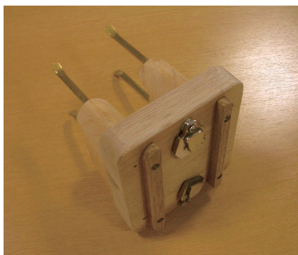
裏面に取り付けた磁石と木枠の様子
